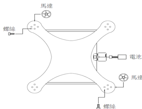
無人機組裝示意圖
